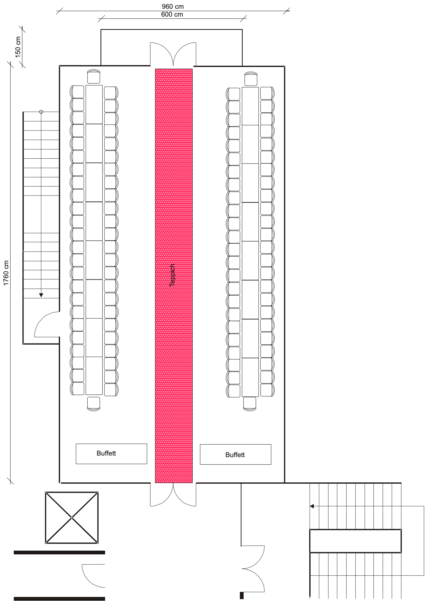
Messe Cottbus Bellevue Beratung 100 Plätze M 1 : 100
