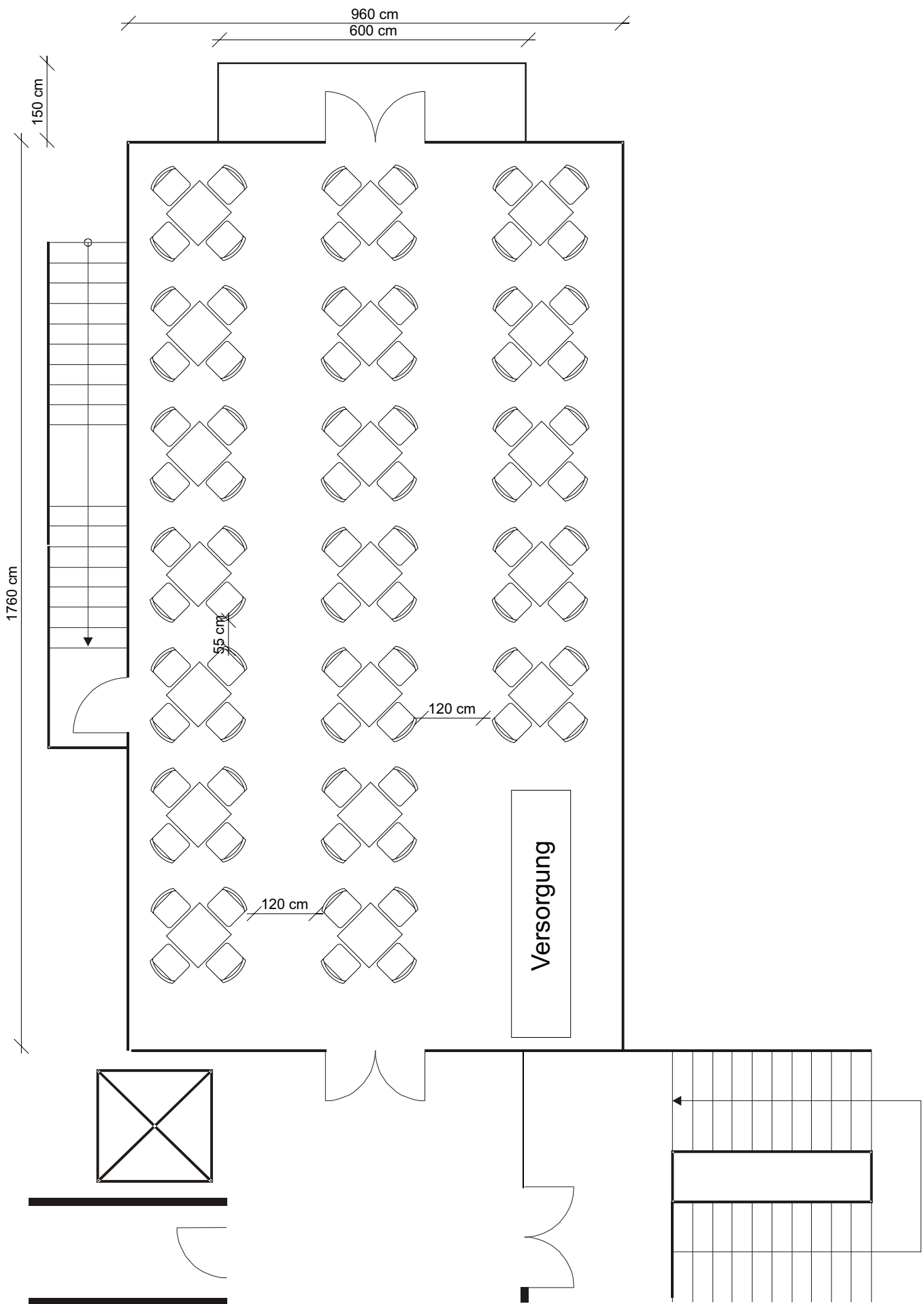
Messe Cottbus Bellevue Gesellsch. 76 Plätze M 1 : 100
